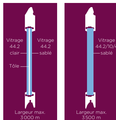
Vitrage + tôle
